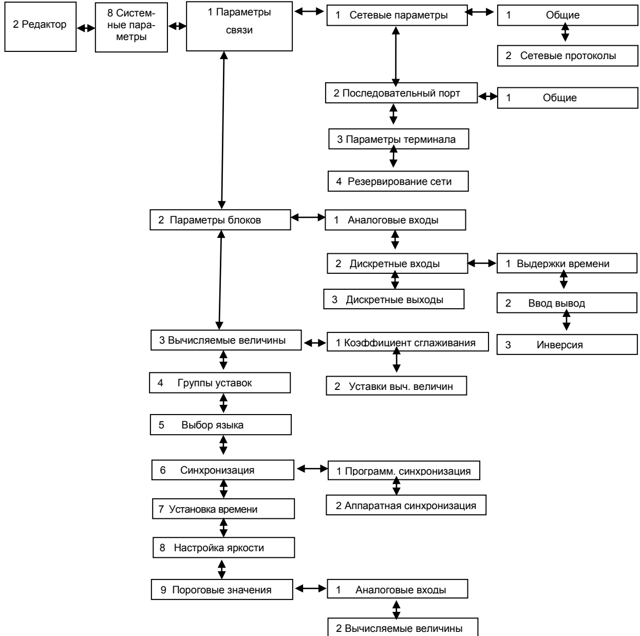
Рисунок 32 – Структура меню Системные параметры
