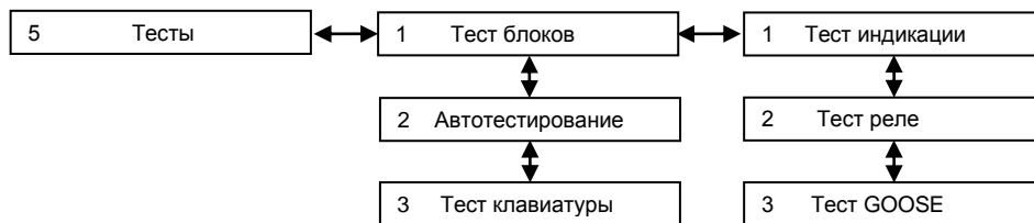
Рисунок 58 – Структура пункта меню Тесты
