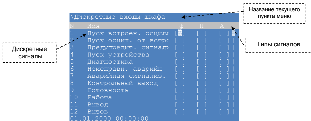
Рисунок 26 – Содержимое пункта меню Дискретные входы шкафа
