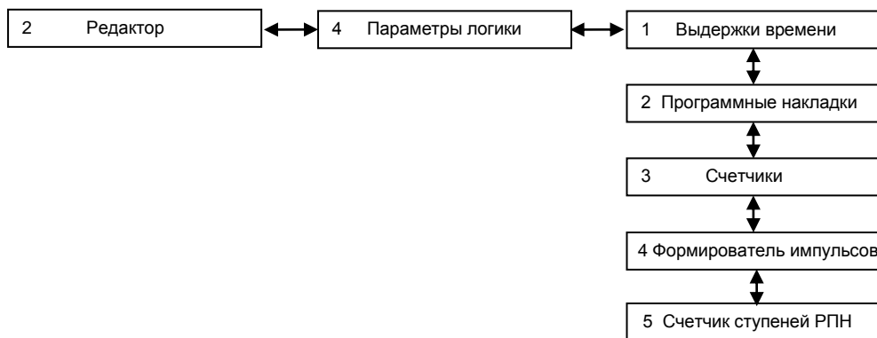
Рисунок 6 – Структура пункта меню Параметры логики
