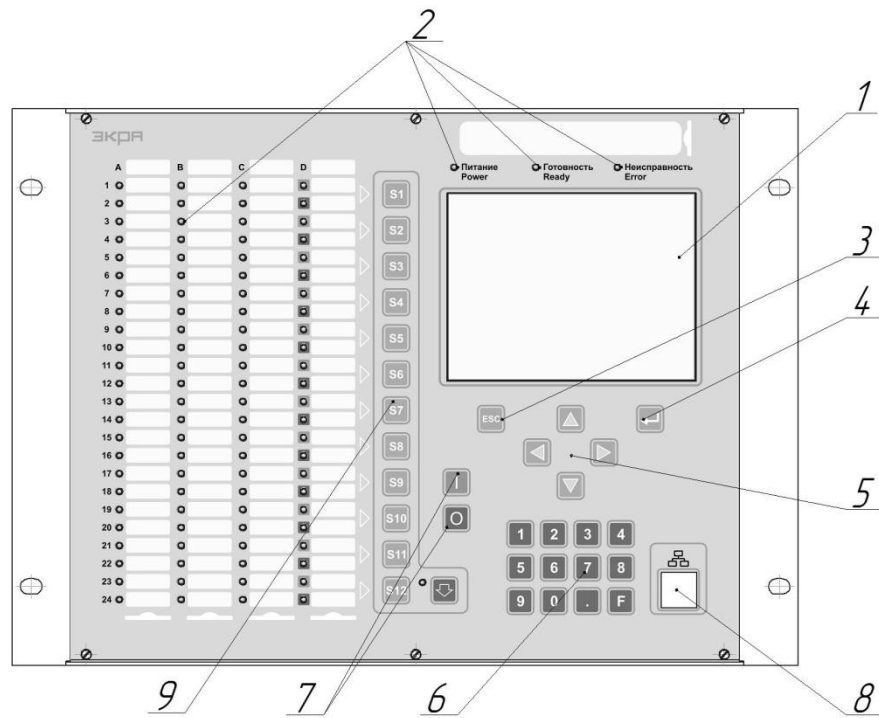
а) терминал типа ЭКРА 2Х2(А)
