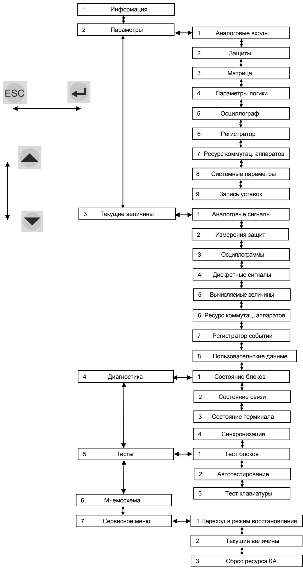
Рисунок 20 – Структура меню терминала с горизонтальным расположением дисплея
