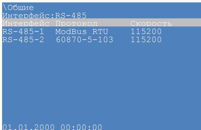
Рисунок 34 – Содержимое пункта меню Общие
