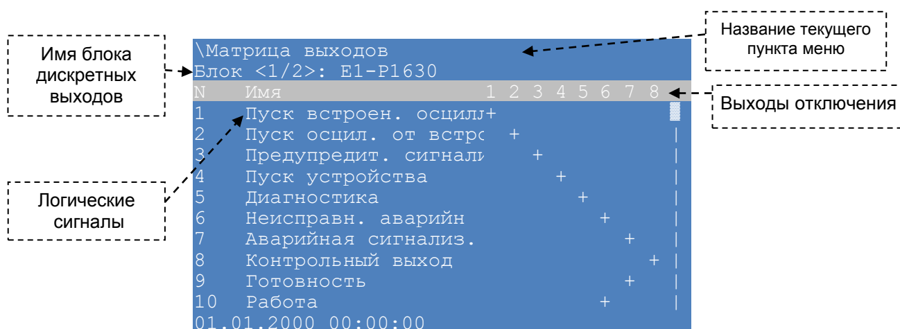
Рисунок 25 – Содержимое пункта меню Матрица выходов
