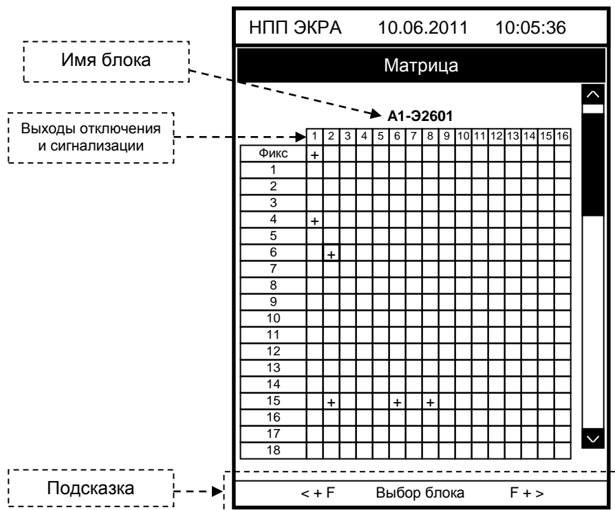
Рисунок 5 – Содержимое пункта меню Редактор матрицы
