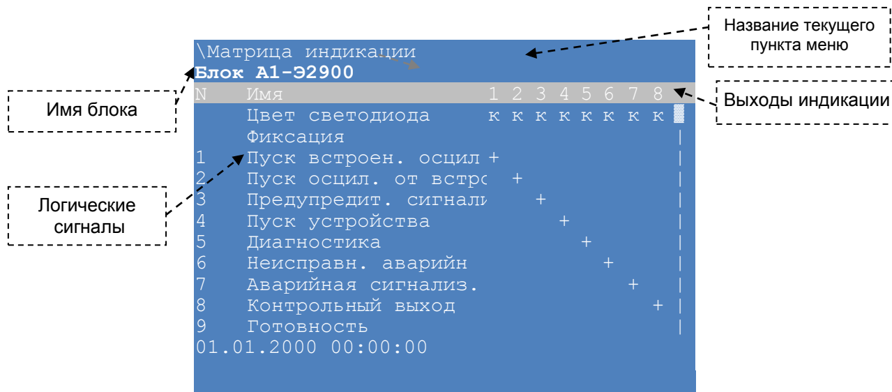
Рисунок 24 – Содержимое пункта меню Матрица индикации
