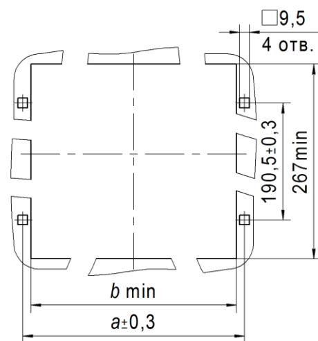
Установочные размеры на месте монтажа
