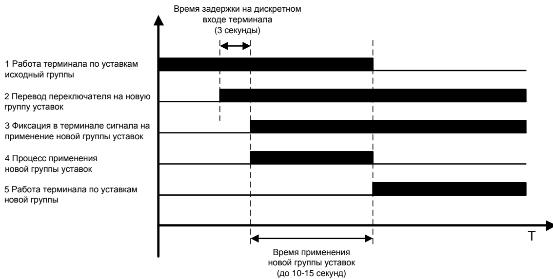
Рисунок 42 – Переключение группы уставок в соседнее положение
