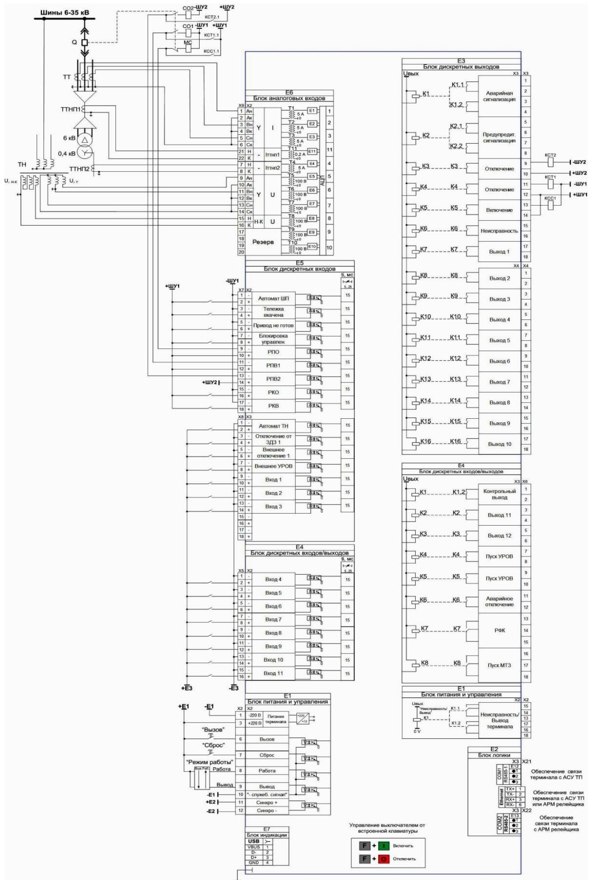
Рисунок 69 – Пример подключения внешних цепей к терминалу защиты кабельной или воздушной линии, линии к ТСН
