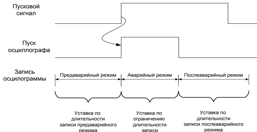
Рисунок 1 – Диаграмма формирования осциллограммы при длительном пусковом сигнале
