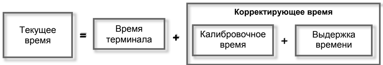
Рисунок 48 – Текущее время терминала (импульсная синхронизация PPS)
