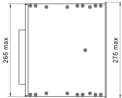
Установочные размеры на месте монтажа
