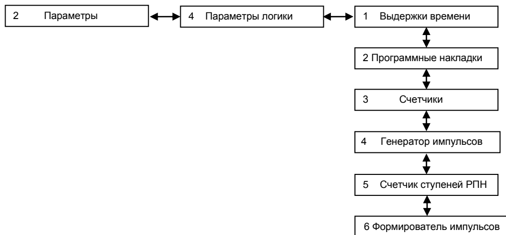
Рисунок 27 – Структура меню Параметры логики
