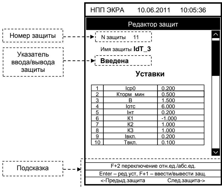
Рисунок 4 – Содержимое пункта меню Редактор защит
