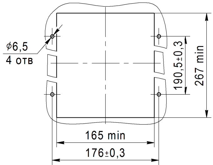
Установочные размеры на месте монтажа
