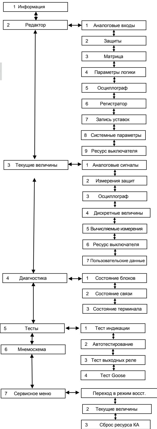
Рисунок 3 – Структура меню терминала с вертикальным расположением дисплея
