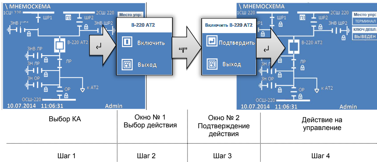
Рисунок 61 – Пример управления выключателем
